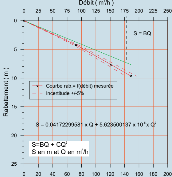
COURBE CARACTERISTIQUE
