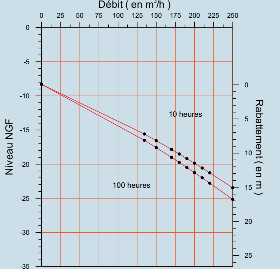
COURBE CARACTERISTIQUE
